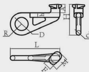
GANCHO DE SEGURANÇA PARA CONTENTORES JAGUAR G.80 TIPO ESQUERDO A 45°
