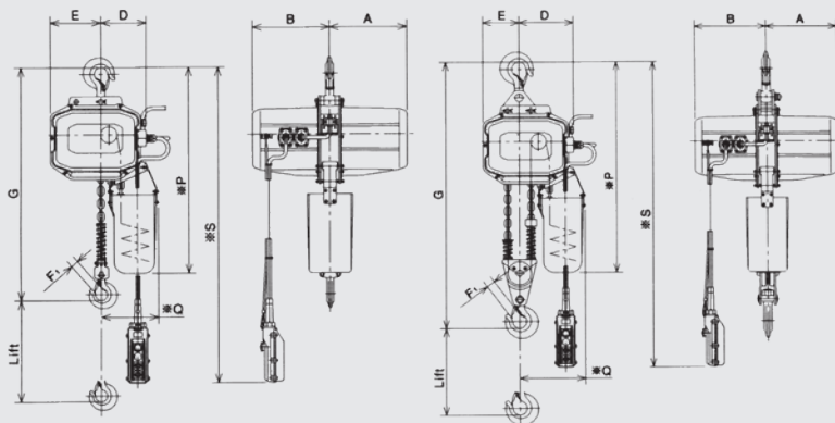
ECT4 · 250 Kg. - 1.000 Kg. (schematic only)
