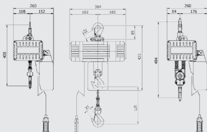
COMPACT - 024 (schématique seulement)
