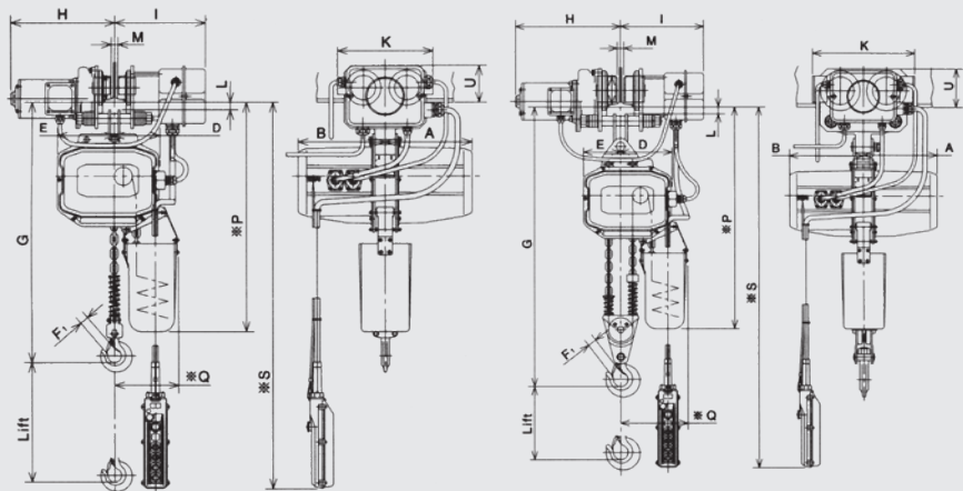
ECEH4 - 500 Kg. - 1.000 Kg. (schematic only)
