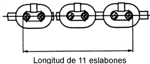
Dimensiones de las cadena de carga (11 eslabones de dimensión)
