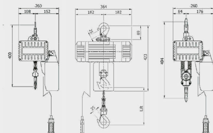
COMPACT - 024 (apenas esquemático)
