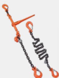
MODELO SPTG E SATC SISTEMAS DE AMARRAÇÃO DE CORRENTE DE GRAU 80
