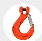
GANCHO COM TRINCO LIGAÇÃO DIRETA MODELO G.80 Pág. 85
