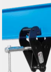
MODELO BCN PINÇA DE ANCORAGEM PARA ESPETÁCULOS
